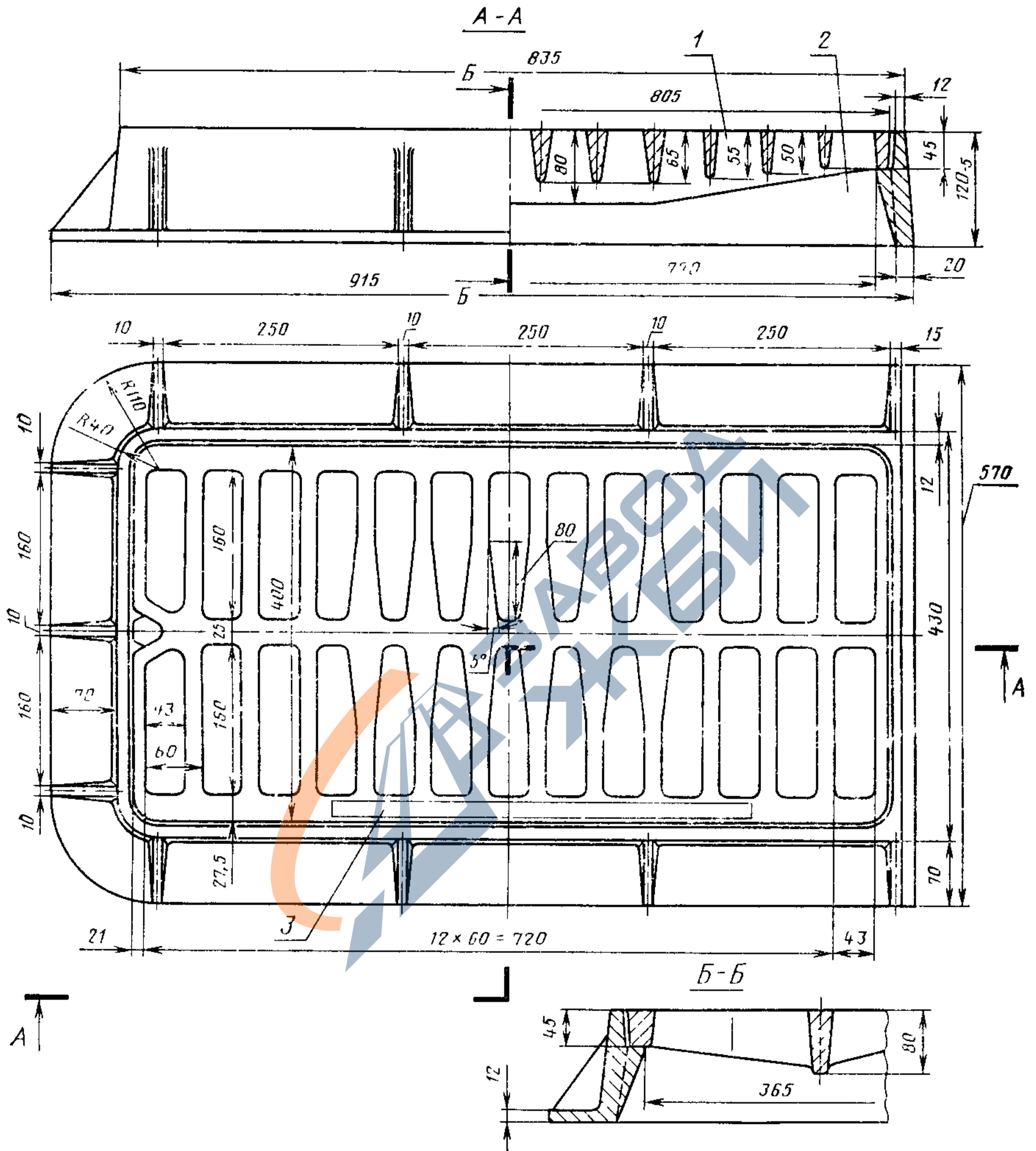
1 — решетка; 2 — корпус; 3 — обозначение настоящего стандарта, тип дождеприемника, год выпуска и товарный знак
